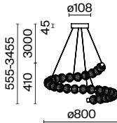
5 MOD555PL-L35G3K LED 40Вт 1900лм t° 3000K >80Ra 360° IP 20
