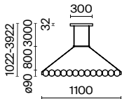
3 MOD555PL-L18G3K LED 22Вт 1050лм t° 3000K >80Ra 360° IP 20
